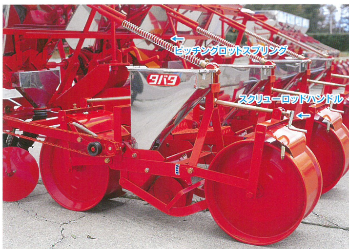
▲ 播種深さは、スクリュローッドにより前後鎮圧ローラーが同時に上下し、地面に対し常に種子箱が平行に上下します。スクリュローッドハンドルで深さの微調節まで簡単にできます。
