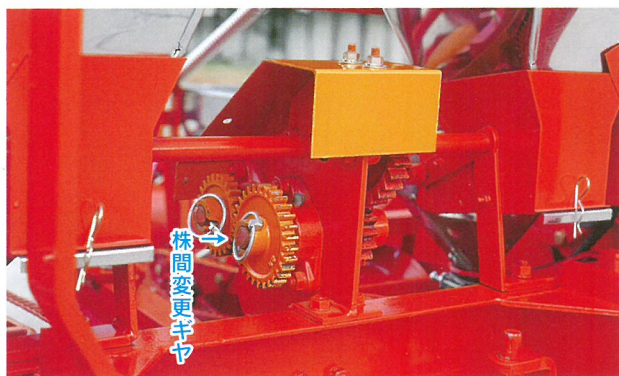
▲ 播種株間は、本機中央ミッションギヤにより全ての播種部株間の調節が一ヶ所でできます。
