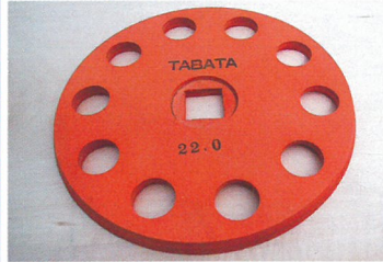
播種板(厚板)
