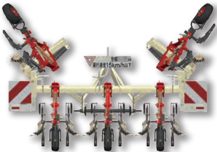
みらくる 草刈るチmid. (NMO-5, NMK-5・7)
