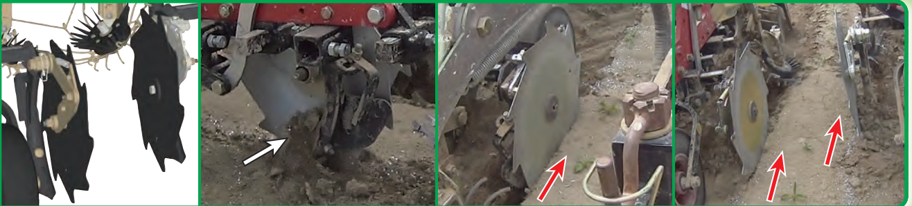
「泥よけシールド」装着
